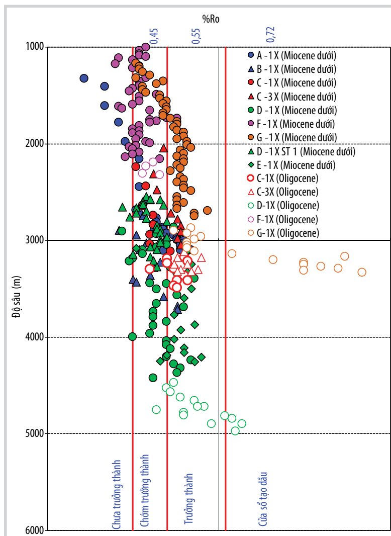
Hình 6. Giá trị phản xạ vitrinite theo độ sâu mẫu từ đáy biển
